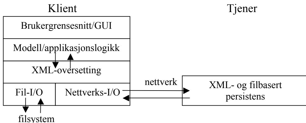
Figur 5 Arkitektur med fil- og nettverksbasert lagring.
