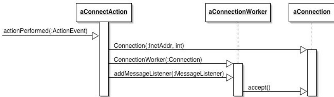
Figur 15 Oppkobling mot en annen kjerneapplikasjon
