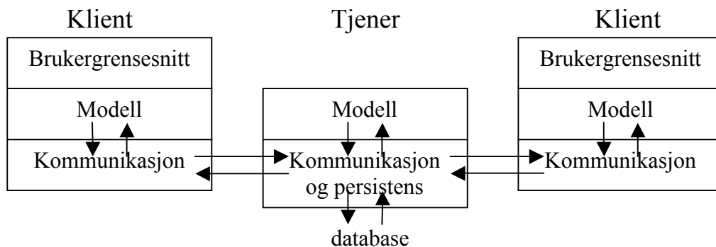
Figur 7 Tjeneren sikrer data vha. databasebasert persistens.
