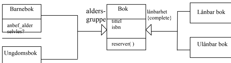
Figur 3: To ortogonale generaliseringshierarkier
