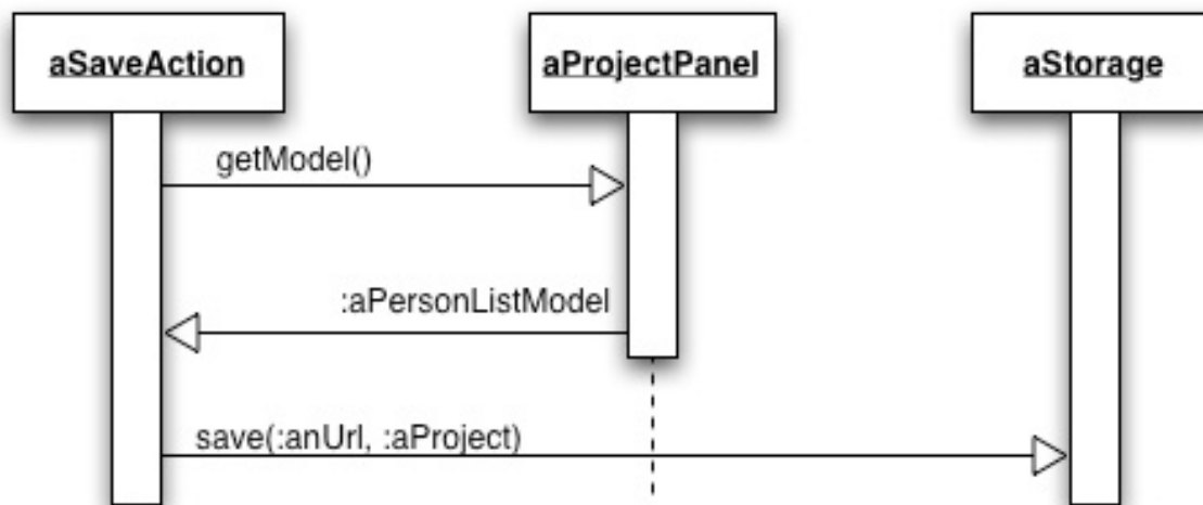
Figur 12 Programsekvensen for å lagre til fil
