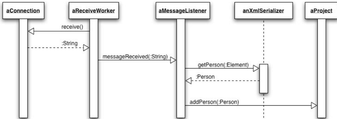
Figur 13 Kjerneapplikasjonen mottar data over nettverket
