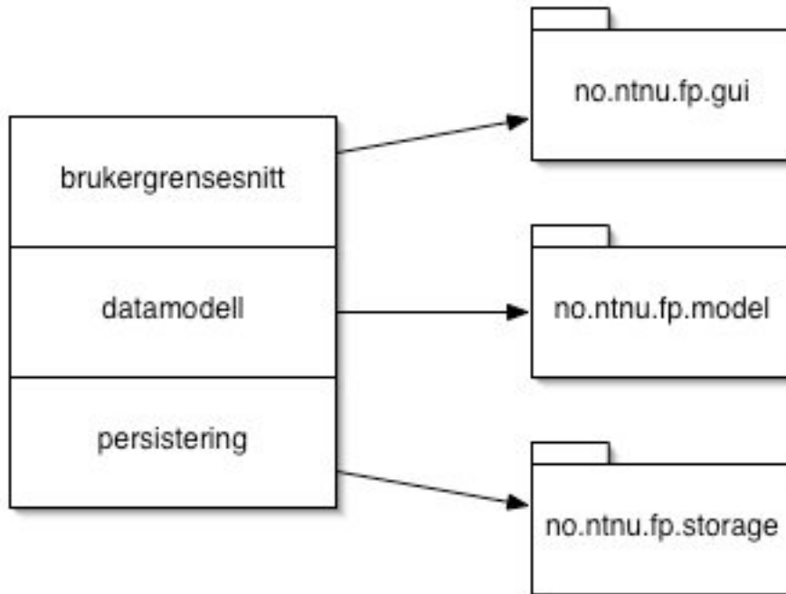
Figur 9 Lagdeling med korresponderende Java-pakker
