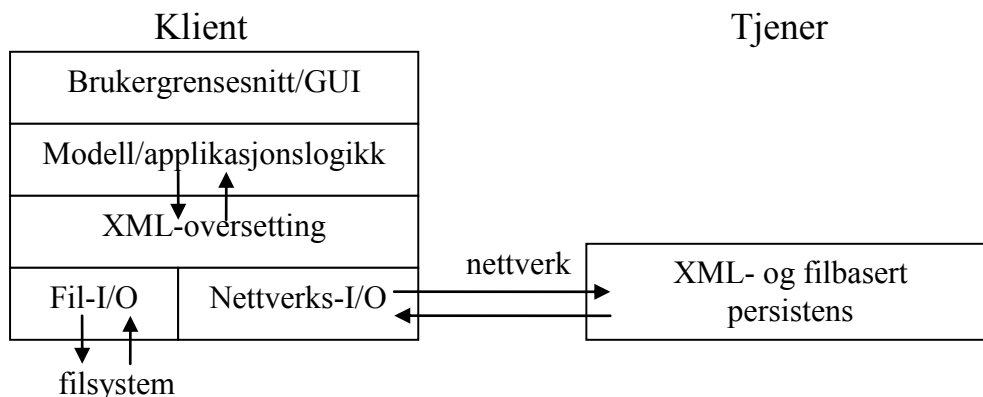
Figur 7 Arkitektur med fil- og nettverksbasert lagring.
