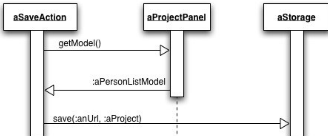
Figur 14 Programsekvensen for å lagre til fil
