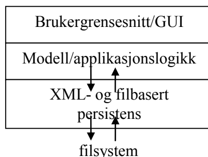
Figur 5 Enkel enbrugerapplikasjon
