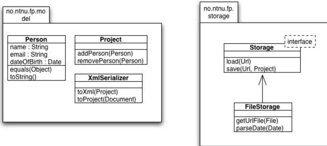
Figur 12 Klassediagram
