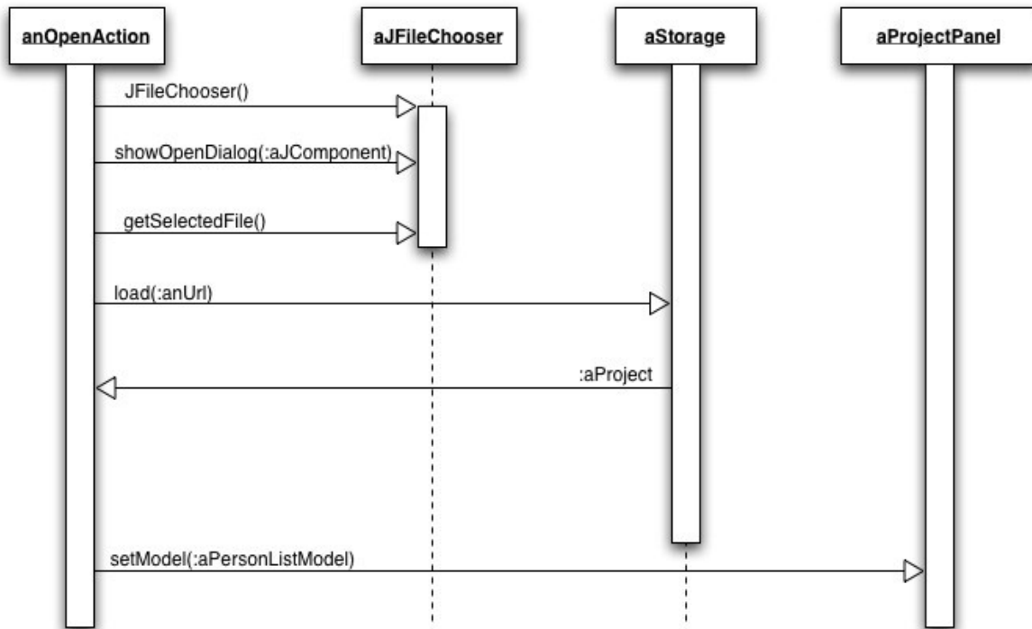
Figur 13 Sekvensdiagram for åpne fil
