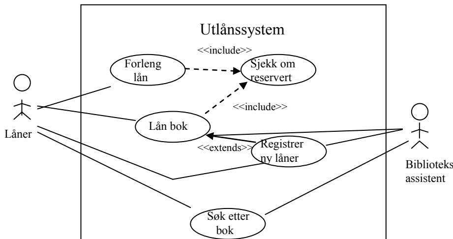
Figur 1: Brukstilfellediagram
