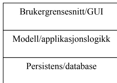
Figur 4 Trelagsapplikasjon
